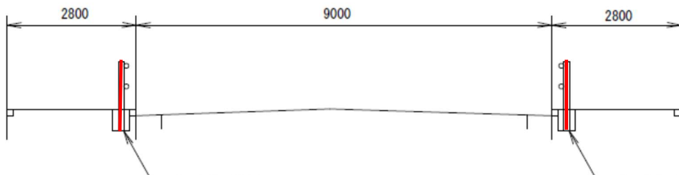
標準横断面図 (1/100)
