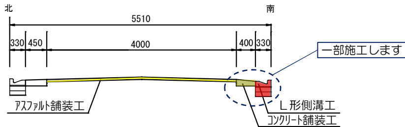
断面図②
